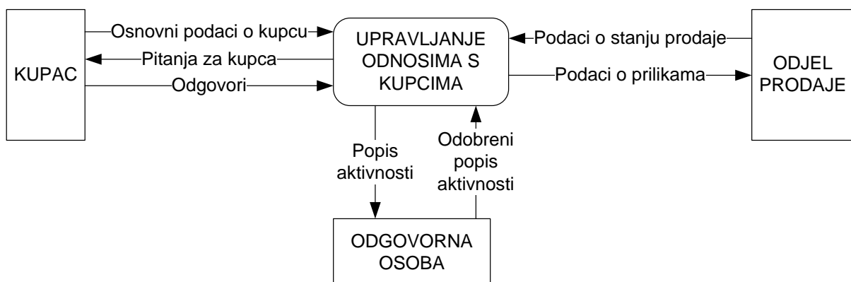
Slika 97: Rješenje zadatka 18 – dijagram konteksta (izvor: Autori)
