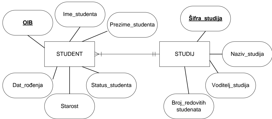
Slika 28: Odnos tipova entiteta "Student" i "Studij" (izvor: Autori)
