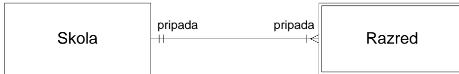
Slika 33: Primjer egzistencijalno i identifikacijski slabog entiteta na EVA modelu (izvor: Autori)
