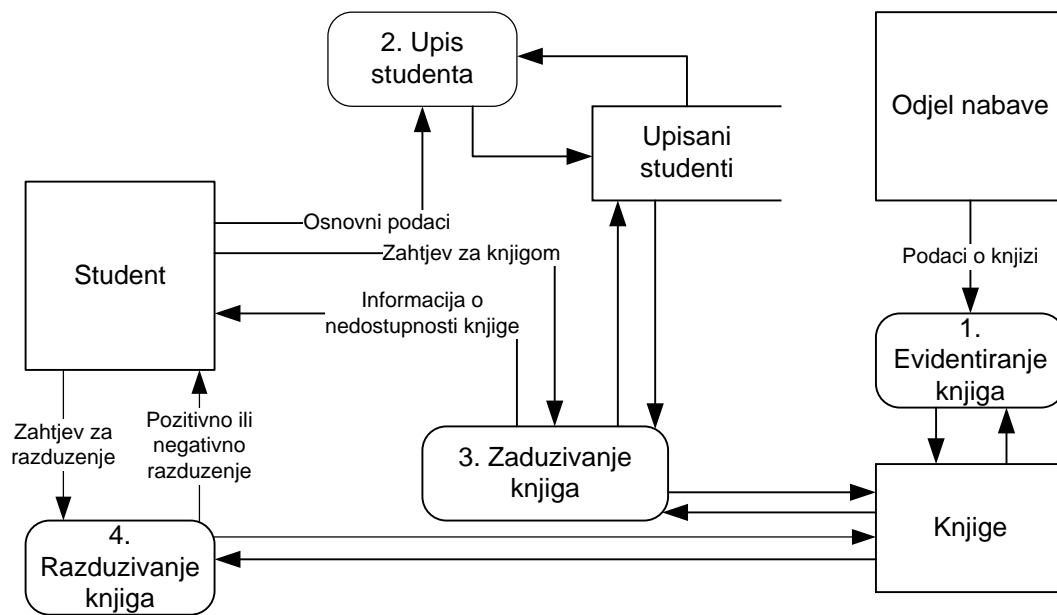
Slika 92: Rješenje zadatka 16 – dijagram 1. razine (izvor: Autori)
