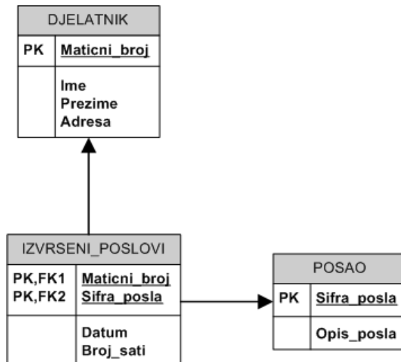
Slika 84: Rješenje zadatka 13 - relacijski model (izvor: Autori)
