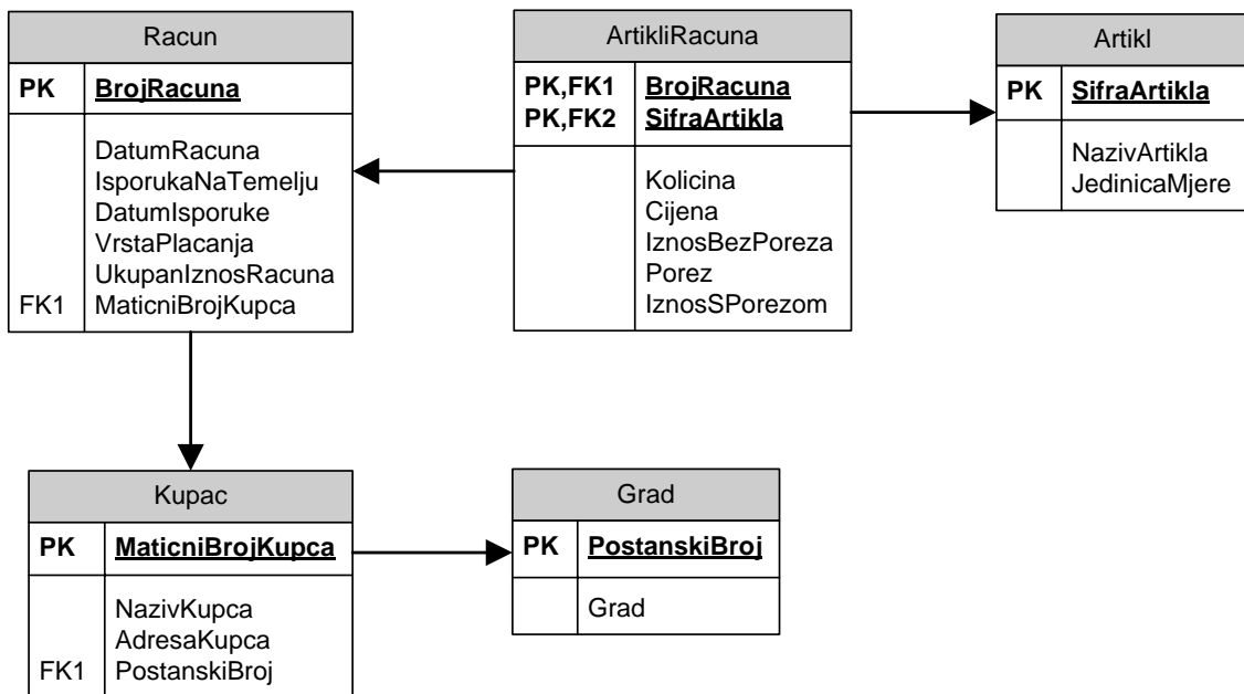
Slika 55: Primjer relacijskog modela podataka (izvor: Autori)
