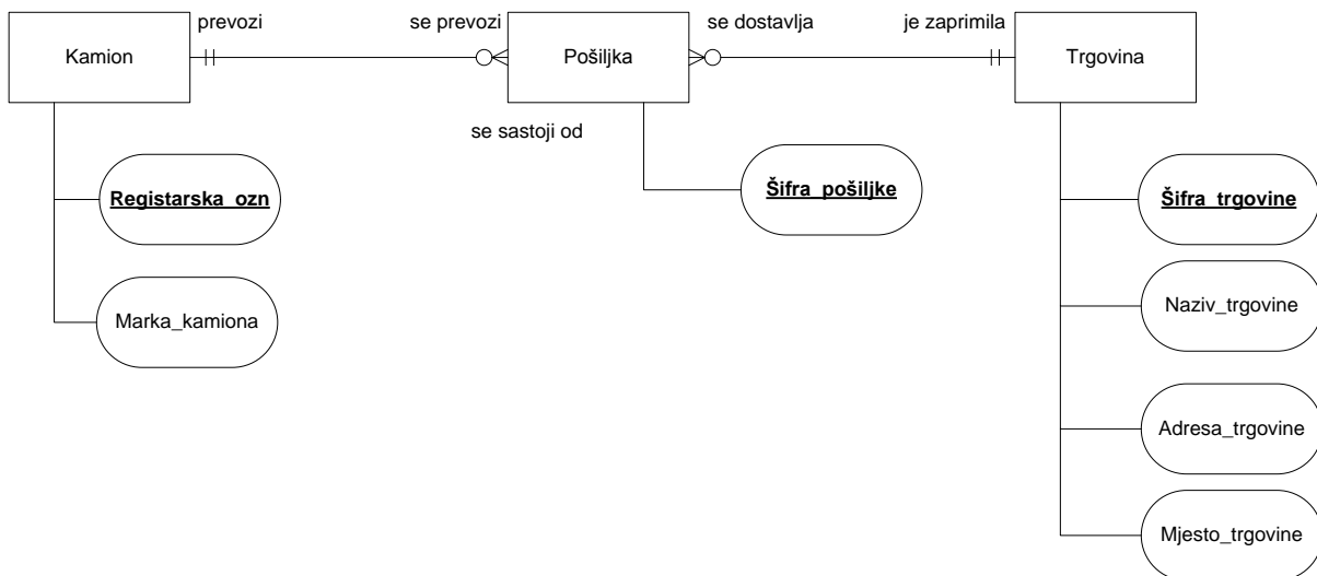
Slika 41: EVA model s vezama 1:M po gornjim granicama (izvor: Autori)
